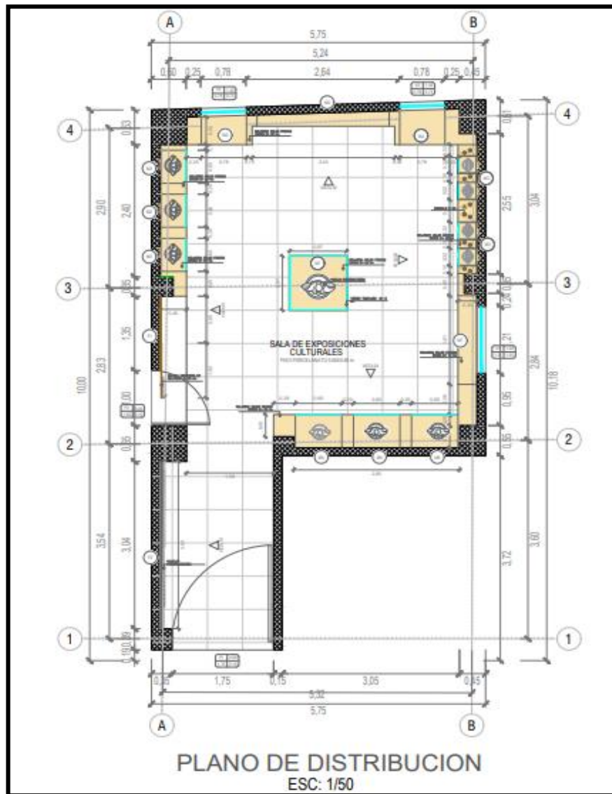
Figura 2: Plano de distribución del salón museográfico. Fuente: Arq. Brandon Santamaria
