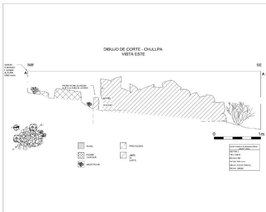
Fig. 77. Corte A-A1 de la Chullpa (Ec-4/SII). Ver el dibujo de planta en la Fig. 76.
