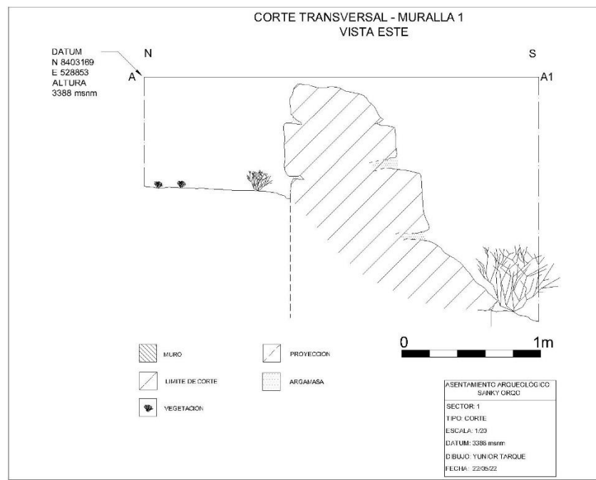
Fig. 39. Corte transversal A-A1 de la Muralla 1. Vista de oeste a este.
