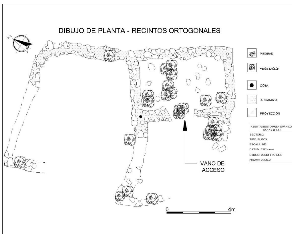
Fig. 90. Dibujo en planta de los Recintos ortogonales (Ec-6/SII).
