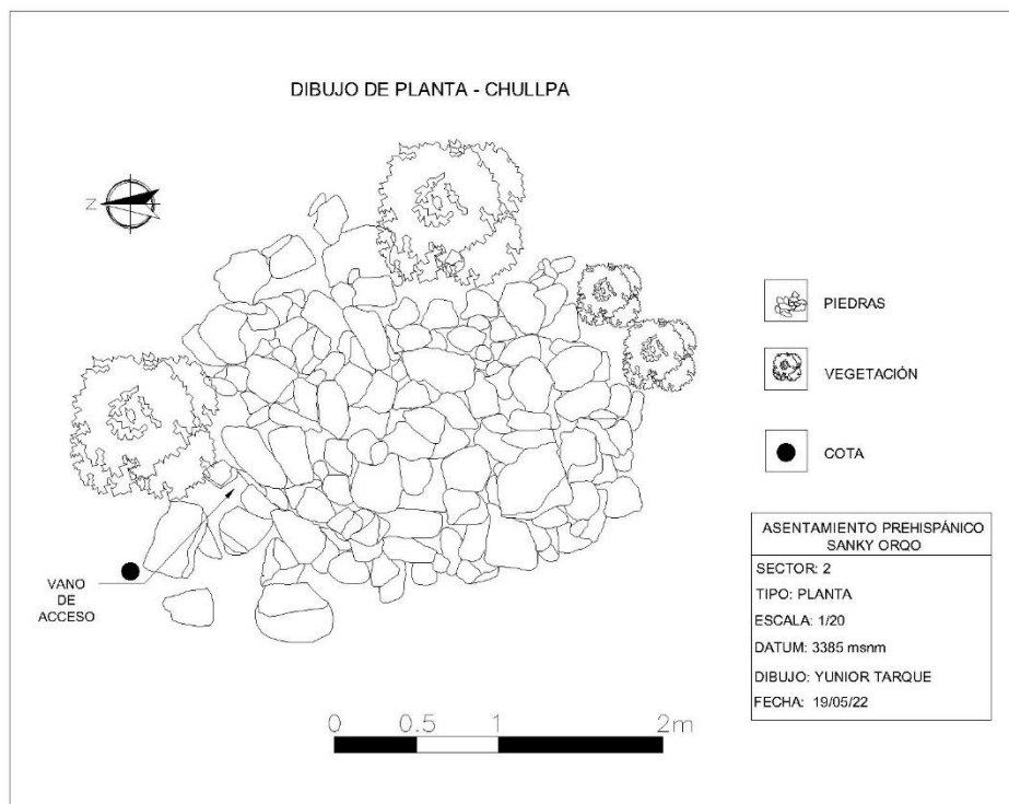
Fig. 76. Dibujo de planta de la Chullpa (Ec-4/SII). Ver el dibujo de corte en la Fig. 77.
