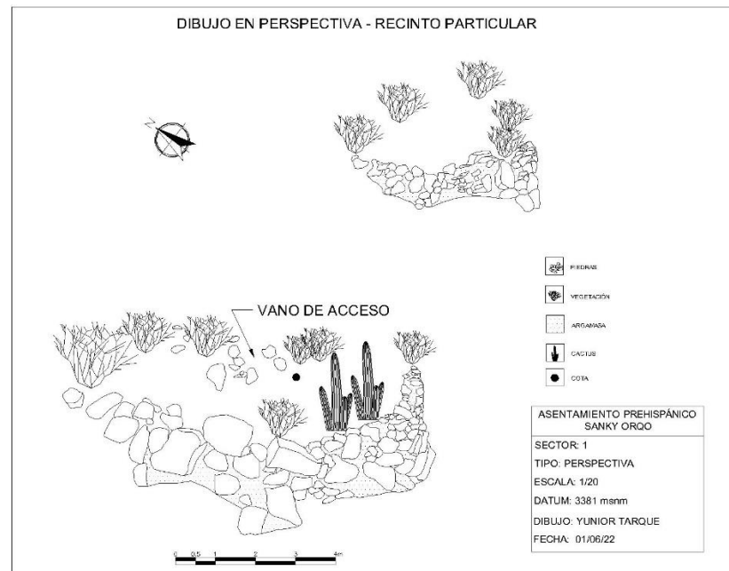
Fig. 24. Dibujo en perspectiva Recinto particular (Ec-4/SI).
