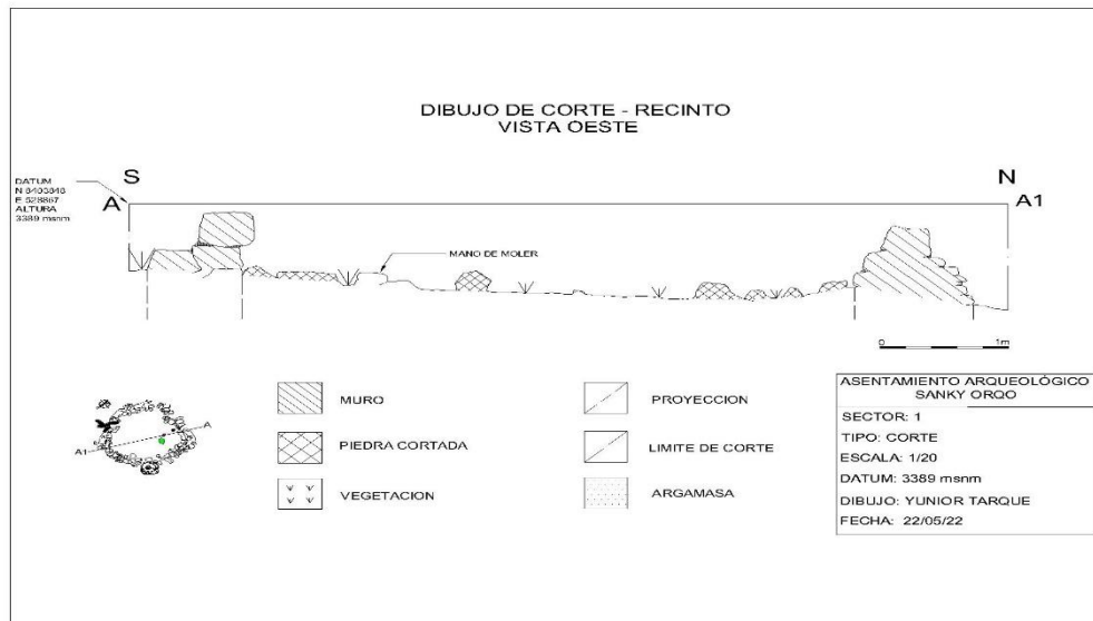
Fig. 14. Corte A-A1 del recinto-muestra del Barrio norte (Ec-2/SI). Véase el dibujo en planta en la Fig. 13.
