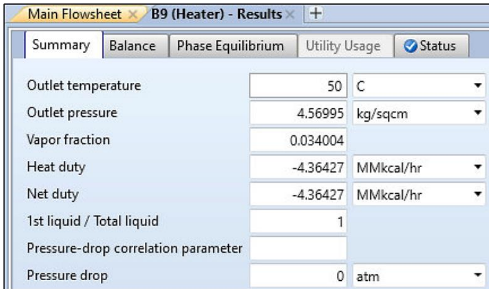
Fig. 41 Condiciones de operación intercambiador de calor B9
