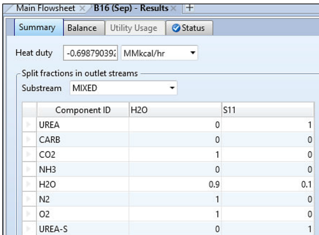
Fig. 42 Condiciones de operación del separador flash de baja presión
